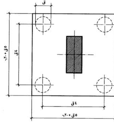
سمك الوسادة من 9-10 سم الوسادة فوق 4 خوازيق
