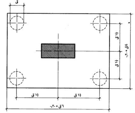
الوسادة فوق 4 خوازيق
