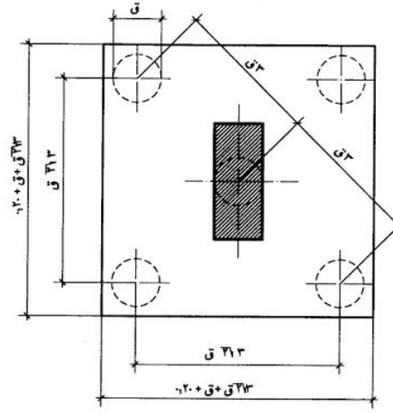
سمك الوسادة من 10-11 سم الوسادة فوق 5 خوازيق
