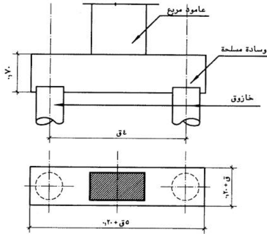
الوسادة فوق خازوقين
