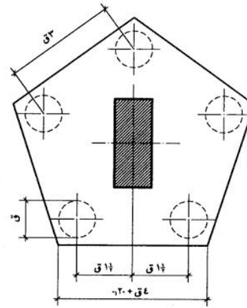
سمك الوسادة من 10-11 سم الوسادة فوق 5 خوازيق
