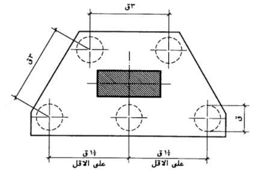
الوسادة فوق 5 خوازيق
