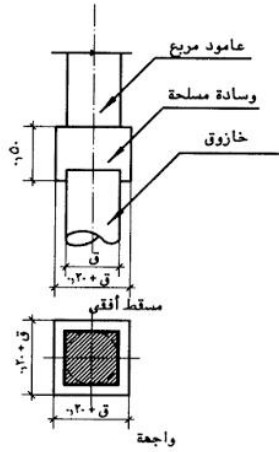
الوسادة لخازوق واحد
